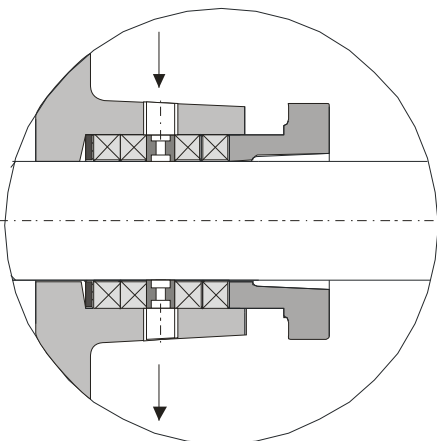
Dławnica sznurowa z płukaniem zewnętrznym
