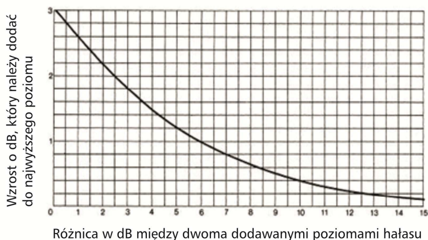
Wykres obliczania wzrostu dB dla dwóch źródeł hałasu
