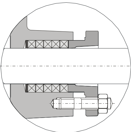
Dławnica sznurowa
