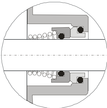
Dławnica mechaniczna podwójna szeregowo (Tandem)
