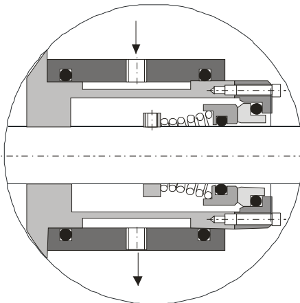
Dławnica mechaniczna podwójna (back to back)
